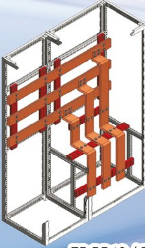
- EB PP 10 / EB PP 25 Uygulama örneği
